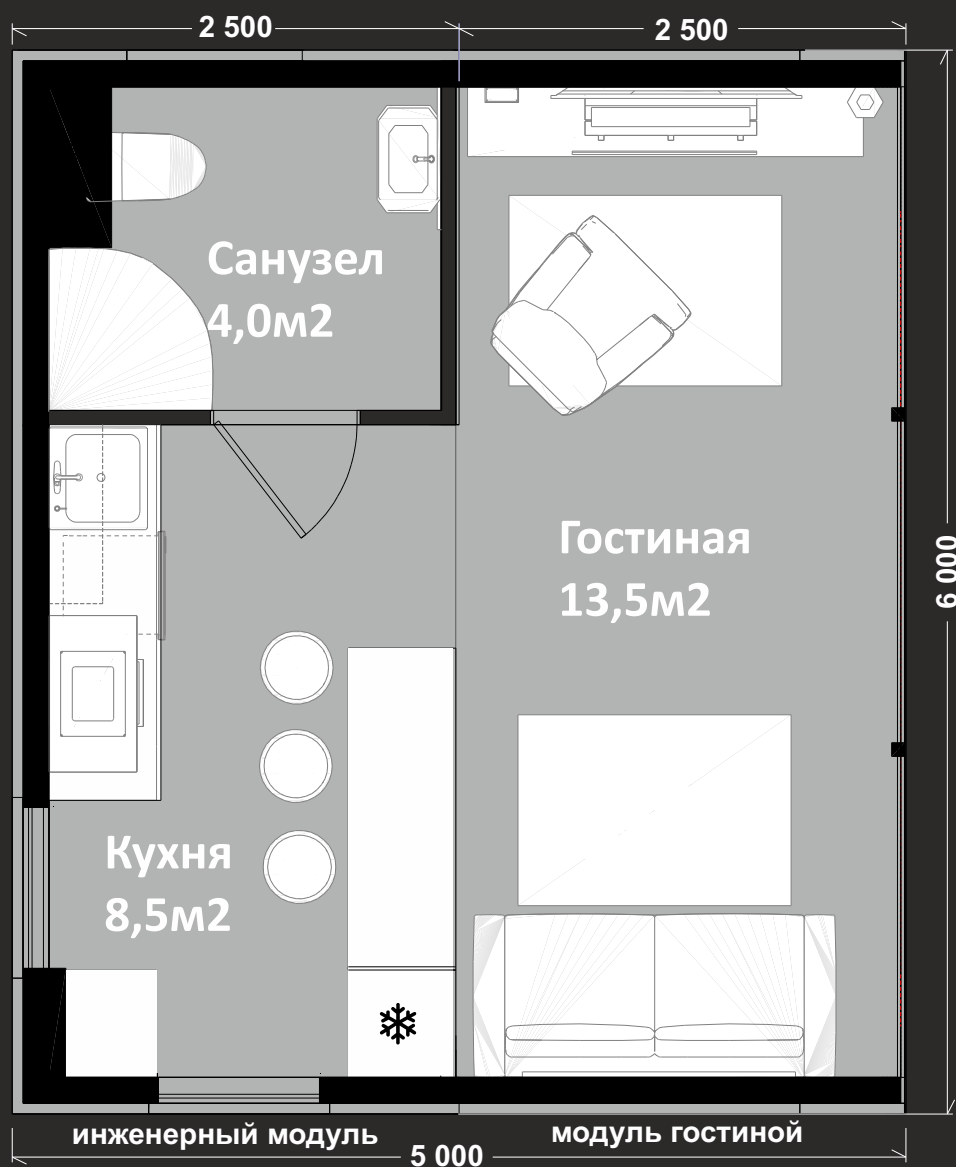
T2-01 - 26м 2 из двух модулей
