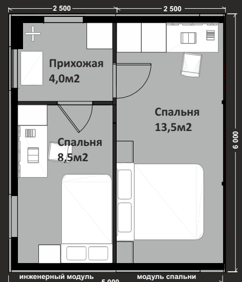
Две спальни Т2-01 - 26м 2 из двух модулей
