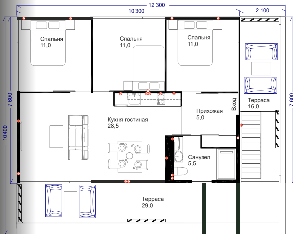
Планировка Smart 7-1 MAX
