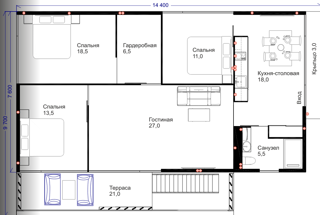
Планировка Smart 9-1 MAX2
