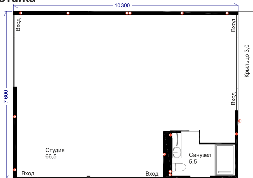
Планировка Smart MAX 0-1
